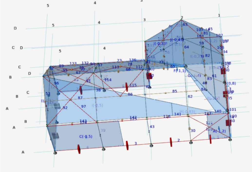
Belastingsgeval : 15 Wind +Y A
